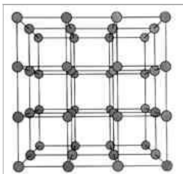
Рис. 12. Кристаллическая решетка
