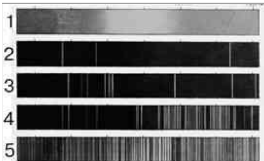
Рис. 4. Виды спектров [1 - непрерывный; 2-4 - линейчатые эмиссионные; 5 - непрерывный спектр Солнца]
