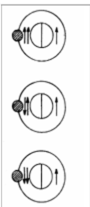
Рис.16. Спины нуклонов в атомах водорода
