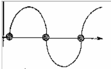
Рис. 2. Модель Вселенной по Фридману
