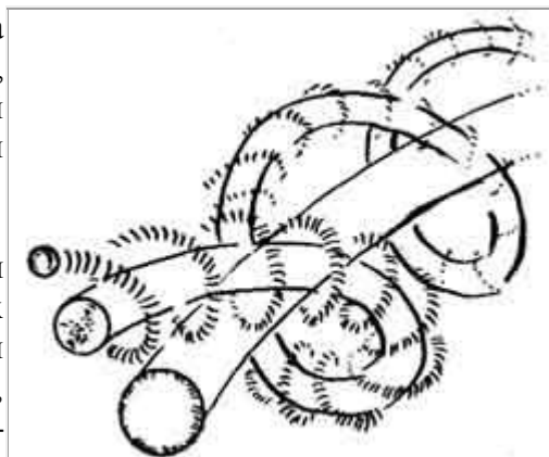
Рис. 25. Солнечная система в четырехмерности: 1 - Луна; 2 - Земля; 3 - Солнце
