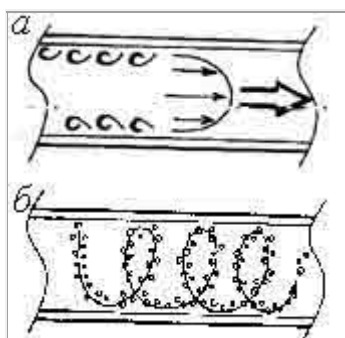
Рис. 41. Прохождение воды в трубе: а-распределение скоростей воды, б-вращение потока воды
